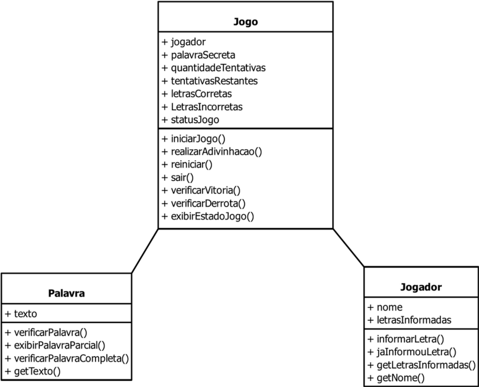
cls Diagrama de Classe
